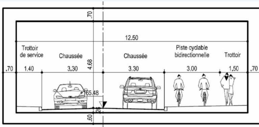
Coupe transversale du passage souterrain créé dans le cadre du projet
